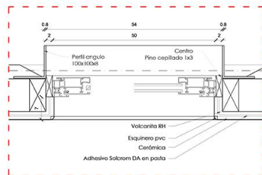
Detalle 2 Escala: 1/5
