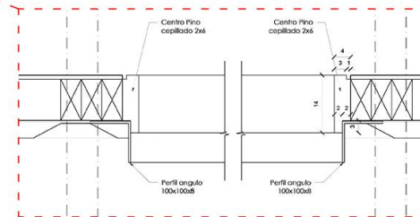
Detalle 5 Escala: 1/5
