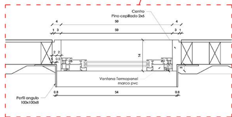
Detalle 7 Escala: 1/5
