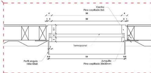
Detalle 6 Escala: 1/5
