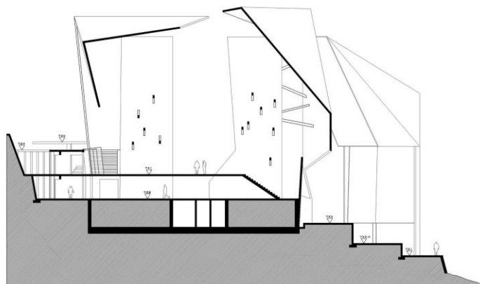
CORTE B-B'
