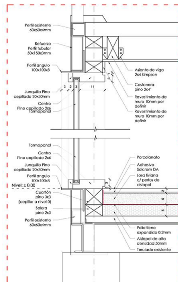
Detalle 10 Escala: 1/5
