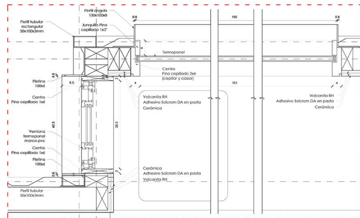
Detalle 3 Escala: 1/5
