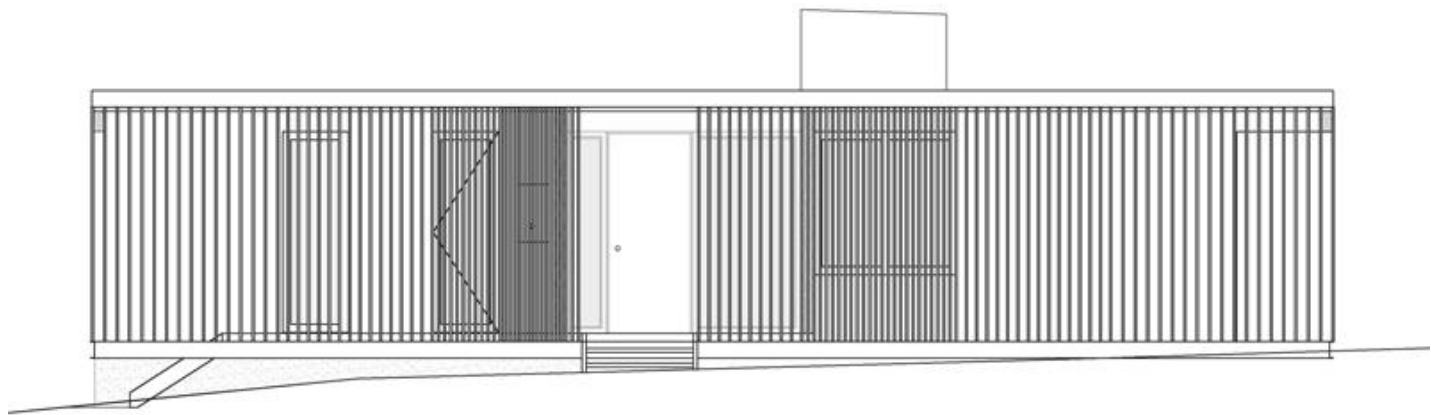
ELEVACION ORIENTE
