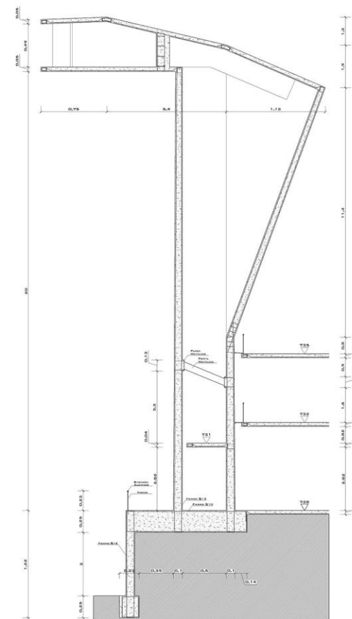
ESCANTILLON
