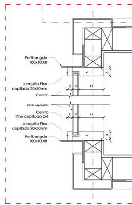
Detalle 1 Escala: 1/5
