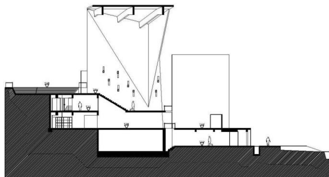
ESCALA 1:100
