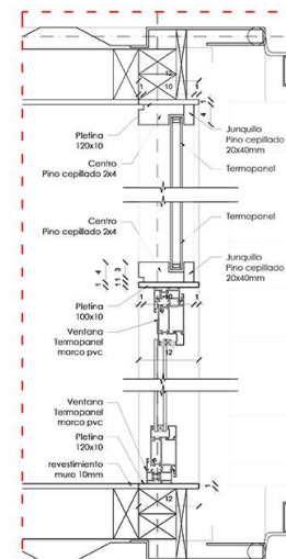
Detalle 4 Escala: 1/5
